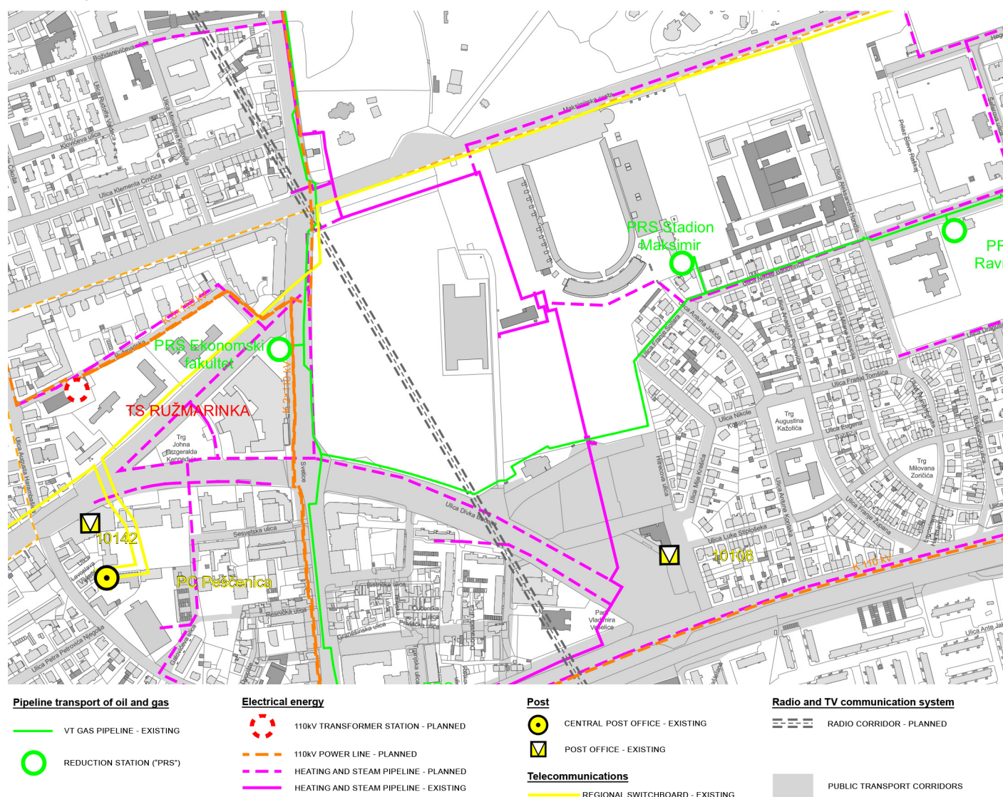
IZVOD IZ KARTOGRAFSKOG PRIKAZA 3 Prometna i komunalna infrastrukturna mreža - 3b. Energetski sustav, pošta i sustav elektroničkih komunikacija
